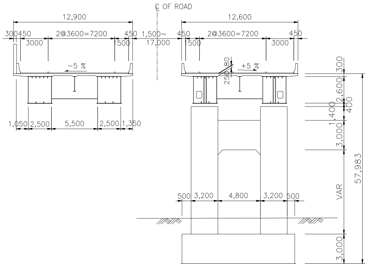
<횡단면도>
